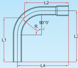
4) Duct 45° / 90° Long Radius Bend
